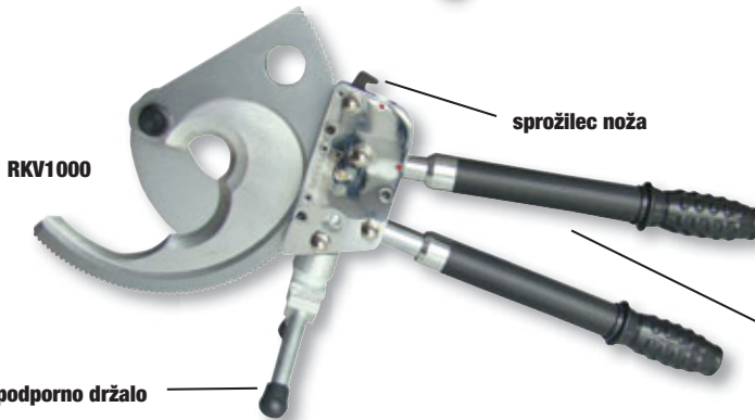
teleskopski ročaj
